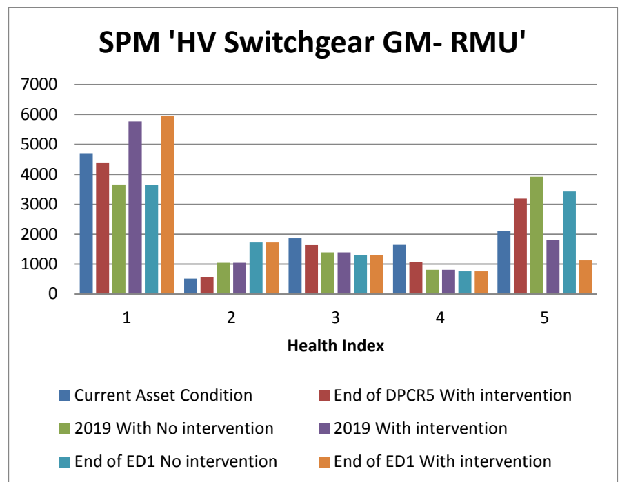
11V RMU
