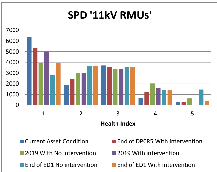
11kV RMU
